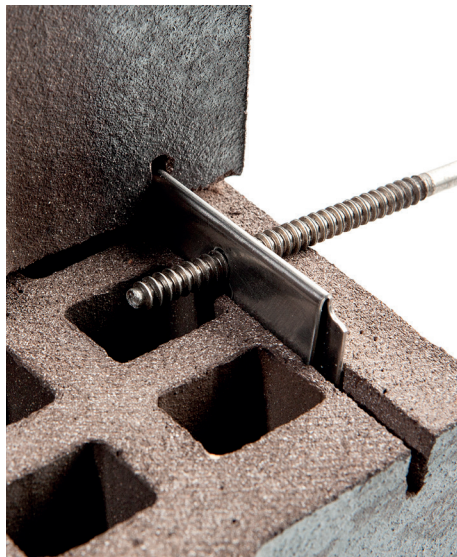
Figuur 51. het ClickBrick systeem
