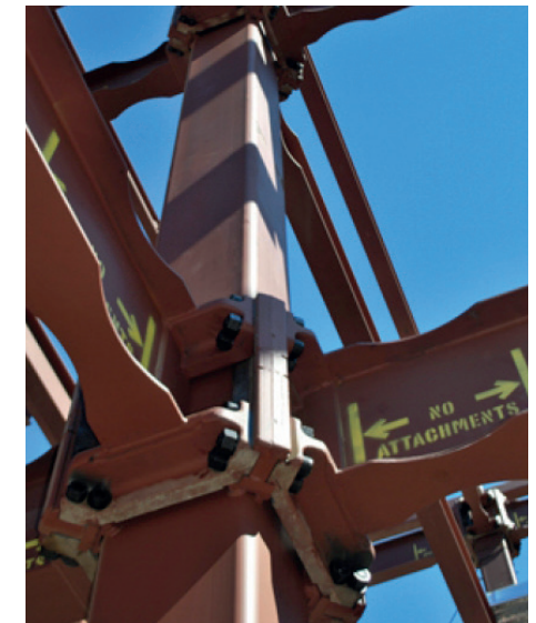
Figuur 44. conXL & conXR
