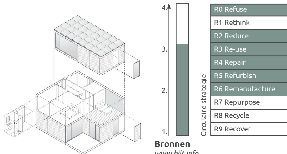
Figuur 83. opbouw BILT woning
